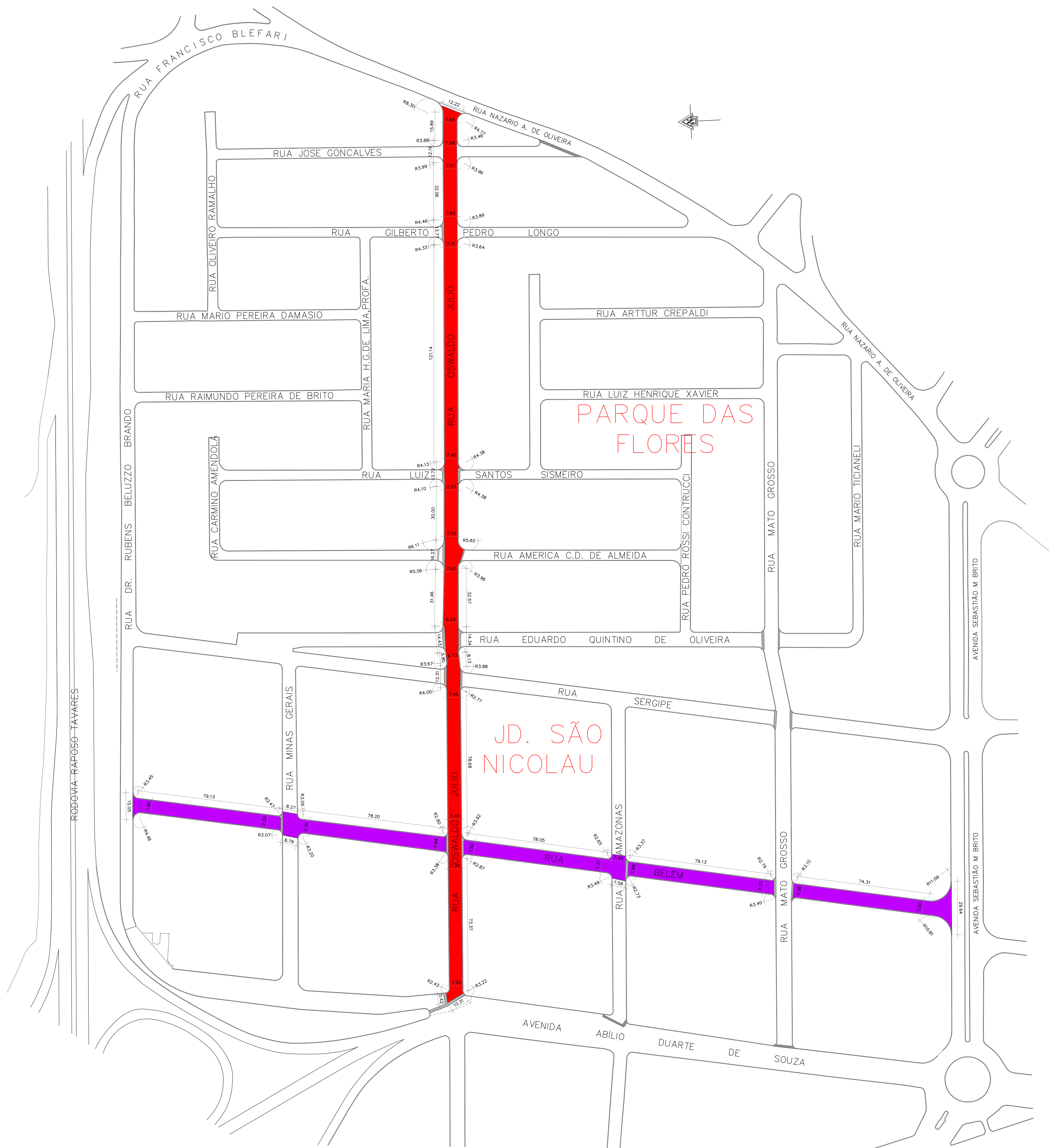
PLANTA DE IMPLANTAÇÃO ESC.: 1:1.000
